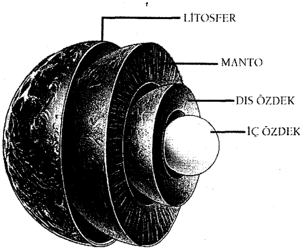
Dünya'nın yarı plastik kayalıklı olan çekirdek ile kabuk arasındaki manto adlı kısmıyla dıştaki katı litosfer, sıvı metalik çekirdekten kesin olarak ayrılır.
