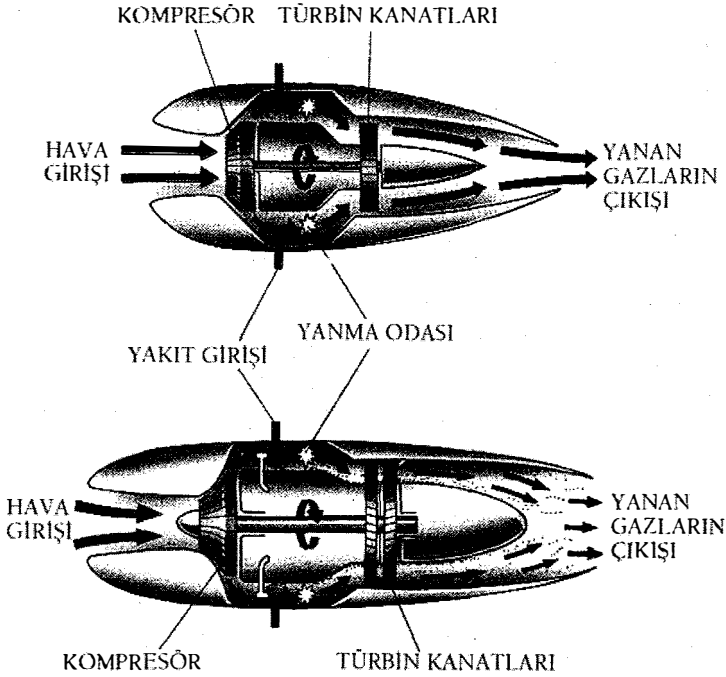
Whittle'in orijinal jet motorunun (yukarıda) öndeki kompresörü çalıştıran tek bir türbini vardı; daha sonraki motorlarda (aşağıda) iki ya da daha fazla türbin kanatları yer aldı.
