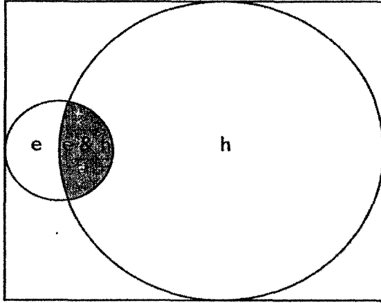
Şekil 10.3 h dairesi e dairesinden çok daha büyüktür, dolayısıyla atılan okun h'ye saplanma olasılığı e'ye saplanma olasılığından çok daha yüksektir. e ile h arasındaki kesişimi gösteren koyu bölge h'den çok küçüktür ve e'nin görece büyük bir oranını oluşturmaktadır. Dolayısıyla p(h/e) yüksektir; p(e/h) ise p(h/e) 'den çok daha düşüktür.
