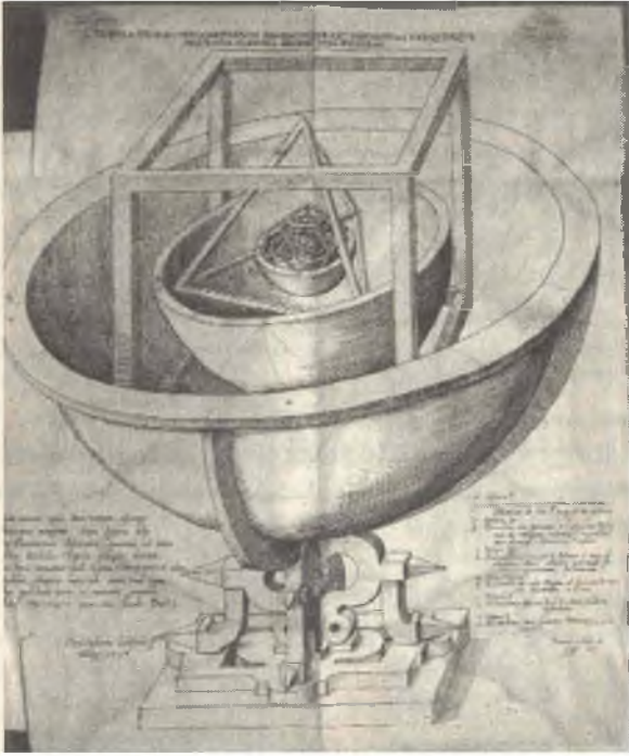
ŞEKİL 16 Kepler'in iç içe gezegenler ve mükemmel cisimler modeli. Johannes Kepler, Mysterium cosmographicum (Evrenin Sırrı, 1596).
