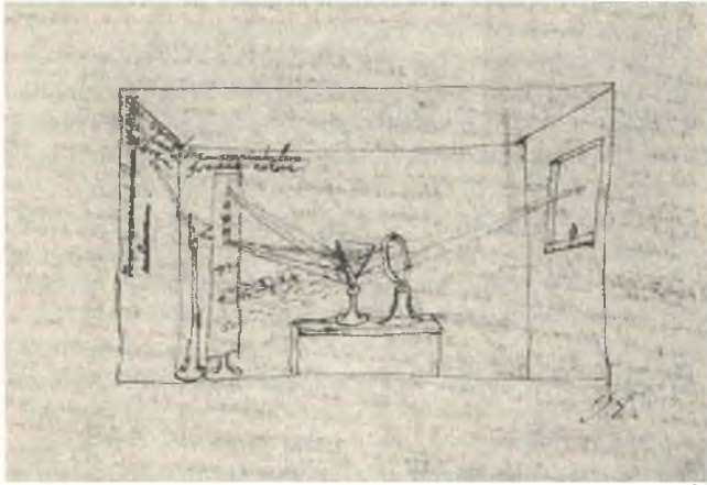
ŞEKİL 21 Isaac Newton'un iki prizmayla yaptığı deneye ilişkin taslağı.
