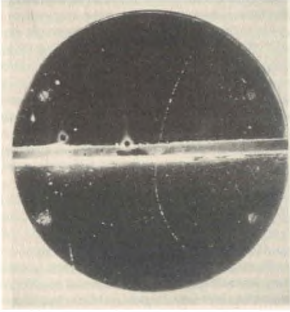
ŞEKİL 45 Carl Anderson'dan ilk pozitron fotoğrafı (1932).
