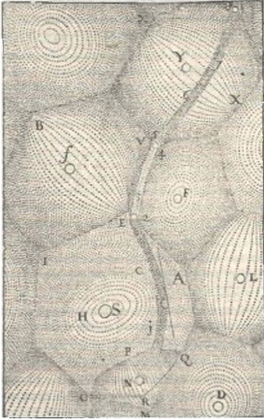
ŞEKİL 18 Descartes'ın gökssel girdaplarının arasında ilerleyen bir kuyruklu yıldızın rotası. René Descartes, Principia Philosophiæ (Felsefenin İlkeleri, 1644).
