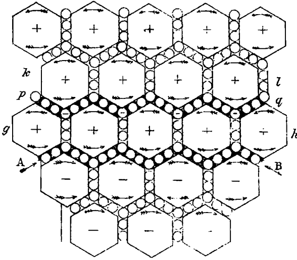
ŞEKİL 39 James Clerk Maxwell'in havayı anlatan fizik modeli. The Scientific Papers of James Clerk Maxwell (James Clerk Maxwell'in Bilimsel Çalışmaları; 1890).
