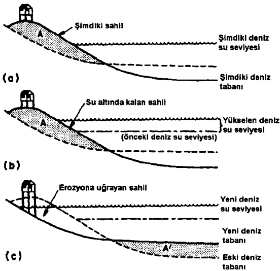
Şekil 4.6. Bruun Kruluna göre deniz suyu seviyesinin yükselmesinin neden olabileceği kıyı erozyonu ve deniz taban yükselmesinin şematik gösterimi. (a) Şu anki sahil, deniz su ve taban seviyeleri (b)'de gösterilen deniz su seviye yükselmesi nedeniyle su basan sahil kesimi (c)'de gösterildiği gibi erozyona uğrayarak deniz tabanını yükseltmektedir (Titus, 1986).
