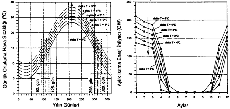
Şekil 5.7. Şeklin sol tarafında değişen hava sıcaklığı ile değişen ısıtma mevsimi başlangıç, bitiş tarihleri ve uzunluklarındaki değişimler gösterilmektedir. Şeklin sağ tarafında da artan hava sıcaklıkları ile birlikte düşen aylık ısıtma enerjisi miktarlarının nasıl değişebileceği gösterilmektedir (Kadıoğlu ve Durmayaz, 2001).
