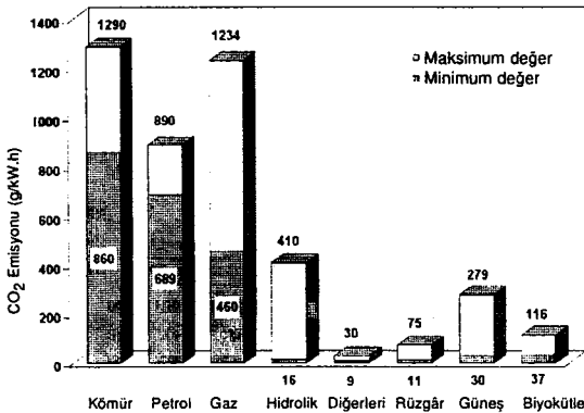
Şekil 5.4. Tüm enerji zinciri için CO 2 eşdeğer emisyonları (IAEA, 1998).
