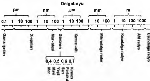
Şekil 1.7. Elektromanyetik spektrum (Durmaz ve Kadioğlu, 2001).
