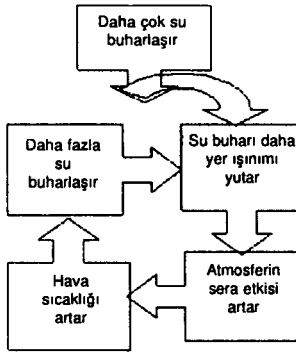
Şekil 4.9. Su buharı-artan sıcaklık (pozitif) geri besleme mekanizması. Küresel ısınma-ya neden olur.
