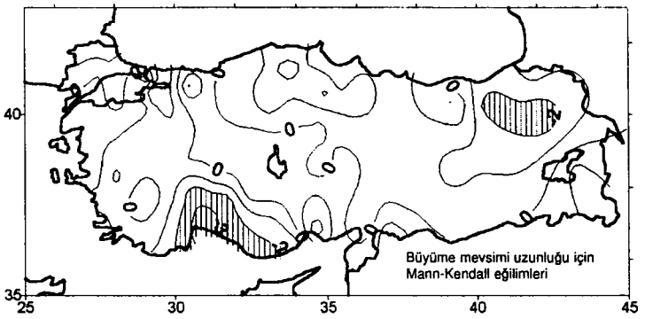
Şekil 5.16. Yıllık ortalama günler olarak verilen yıllık bitki büyüme mevsimi uzunluklarının veri dönemi boyunca nasıl değiştiğine dair Mann-Kendall eğilim istatistiği. (1,96'lık kontur değerleri eğilimlerin %5 seviyesinde önemli olduğunu göstermektedir.)
