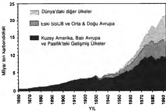
Şekil 5.3. Üç ülke grubu için 1860-1992 yıllarında kömür, petrol ve doğal gazın yanmasından oluşan CO 2 emisyonları (Hamburg ve ark., 1997).
