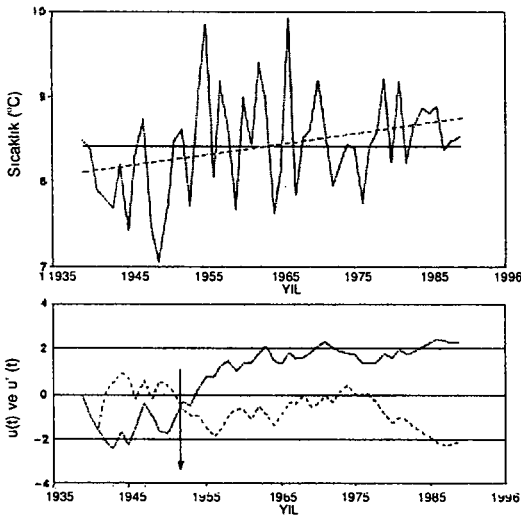
Şekil 5.1. Şeklin üst kısımda Türkiye'nin yıllık ortalama gece (minimum) hava sıcaklıklarının yıllara göre değişimi, doğrusal eğilim hattı (kesikli düz çizgi) ve ortalaması. Alt kısımda ise düz ve kesikli çizgilerinin birleştiği yer, Mann-Kendall eğilim testine göre, önemli trendin başlangıç yılıdır (Kadioğlu, 1997).
