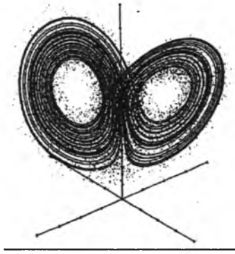
Şekil 1.12. Hava tahmini ile ilişkili olan ve kelebeğin kanatlarına da benzetilen tuhaf çekici. Birbirine çok yakın olan on bin nokta, hava sistemlerinin harekete başlangıç değerlerini göstermektedir (Tsonis ve Elsner, 1989).
