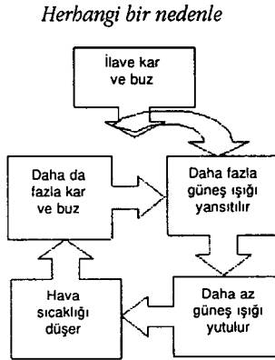
Şekil 4.11. Kar-albedo (negatif) geri besleme mekanizması. Küresel soğumaya neden olur.
