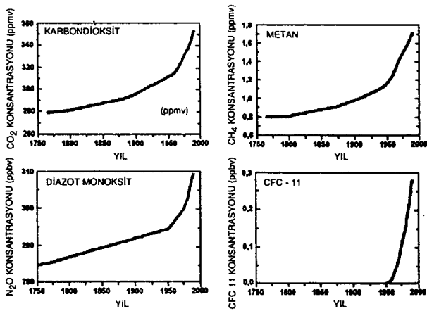
Şekil 4.2. Bazı atmosferik sera gazları konsantrasyonlarının 18. yüzyılın ortalarından itibaren zamanla değişimi (Houghton ve ark., 1990).
