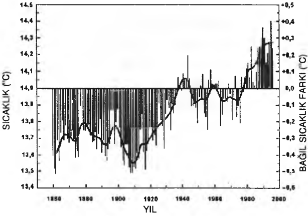
Şekil 4.3. 1860-1996 yılları için yeryüzünde ölçülen küresel ortalama hava sıcaklıkları ve bu sıcaklıkların 1961-1990 yılları için belirlenen sıcaklık ortalamasına nazaran değişimi (Hamburg ve diğ, 1997, Durmayaz ve Kadıoğlu 1999).
