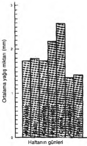
Şekil 3.14. Paris'te 8 yıllık periyotta (1960-1967) ait bir haftalık günler için ortalama yağışlar. Pazartesi'den Cuma gününe kadar yağıştaki giderek artış ve C.tesi ile Pazar günlerindeki keskin düşüşe dikkat edin. Hafta içinde yağışın ortalaması 1,93 mm'yi hafta sonundaki 1,47 mm'lik yağışla karşılaştırm. Aradaki fark % 24'dür. (Derwiller ve Landsberg, 1974).
