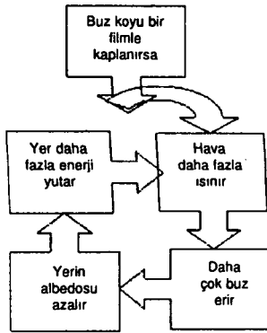
Şekil 4.10. Yapay bir pozitif geri besleme mekanizması ile küresel ısınmanın artırılması.
