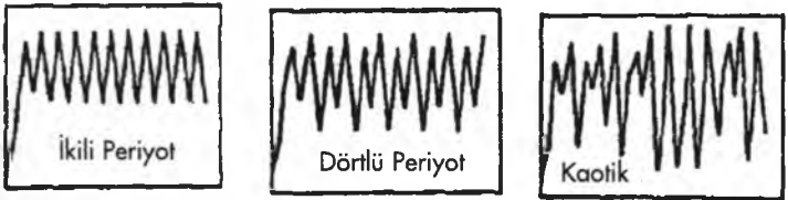
Şekil 2.3. Düzenli ikili ve dörtlü periyodik hareketler ile birlikte kaotik bir davranışın şematik gösterimleri.
