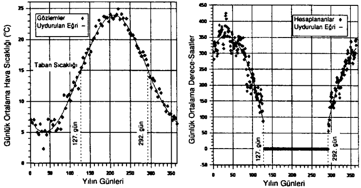
Şekil 5.6. Şeklin solunda İstanbul (Göztepe'de), taban sıcaklığı, günlük ortalama hava sıcaklıklarının yıl içindeki gidişatı verilmiştir. Bu şekilde aynı zamanda İstanbul'daki ısıtma mevsiminin başlangıç ve bitiş tarihleri ile birlikte gösterilmektedir. Şeklin sağ tarafında ise ortalama günlük hava sıcaklıklarına göre ısıtma mevsiminde değişen ortalama derece-saat değerleri gösterilmektedir (Durmayağ ve ark., 2000).
