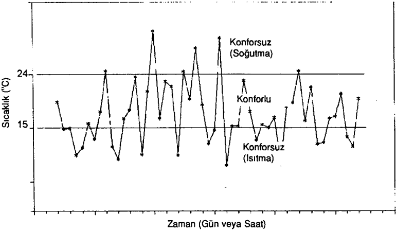
Şekil 5.5. Taban sıcaklığı kavramının şematik gösterimi. Günlük ortalama hava sıcaklığı 15°C çizgisinin altına düştüğünde ısıtma ihtiyacı ortaya çıkar. Benzer şekilde 24°C hattının üstünde kalan hava sıcaklıkları konutların soğutma ihtiyacını doğurur. 15°C ile 24°C arasındaki hava sıcaklıkları insanlar için konforludur. Örneğin 5°C'lik bir hat çizilip üzerinde kalan hava sıcaklıkları dikkate alındığında da bitkilerin büyümesine yönelik genel bilgiler elde edilir.
