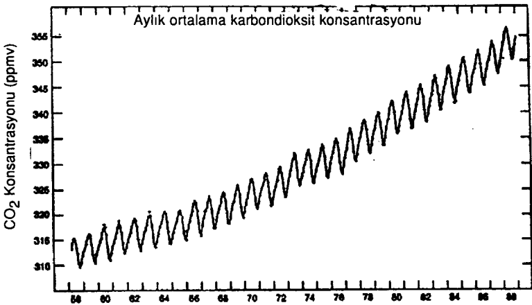
Şekil 4.1. Yapay kirletici kaynaklarından çok uzakta bulunan Hāwāii, Mauna Loa Gözlem evinde gözlenen atmosferik karbondioksit miktarları. 1958 yılından beri atmosferik karbon dioksit miktarında önemli bir artış olduğu görülmektedir. Yıllık salınımlara, vejetasyondaki büyüme ve azalmalar neden olur (Ennis ve Marcus, 1993).
