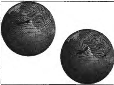
Şekil 2.16. Kış aylarında jet akımı seviyesindeki rüzgârlar (oklar), normal şartlardaki (yukarıdaki şekil) pozisyonundan (aşağıdaki şekilde gösterilen) El Nino yılındaki pozisyonla yer değiştirir. Böylece yukarı seviyedeki hava sirkülasyonu da (Rossby dalgaları vasıtası ile) değişir.
