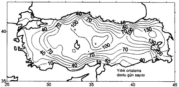
Şekil 5.14. 1961-1990 dönemi 75 meteoroloji istasyonunun en düşük hava sıcaklıkları ve risine göre Türkiye üzerindeki donlu günler sayısının yıllık ortalamaları (Kadioğlu ve Aslan, 2000).
