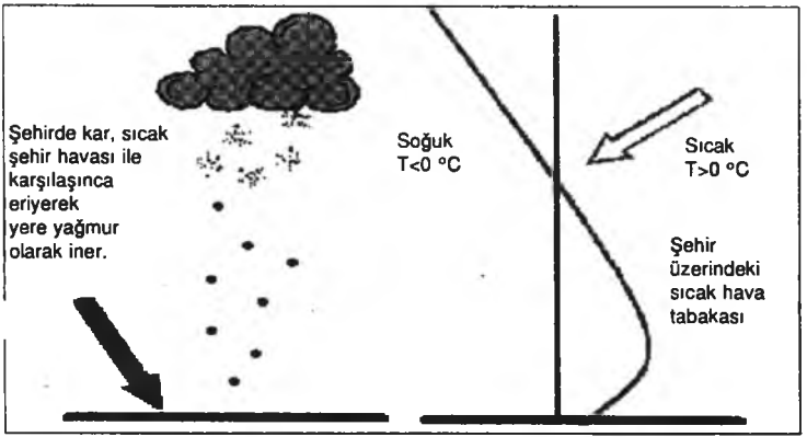
Şekil 3.11. Ülkemizin bulunduğu enlemlerde yağışlar genellikle bulutlardan kar şeklinde başlar. Buluttan düşen kar kristalleri, aşağı seviyedeki hava tabakasının sıcaklığı 0^{\circ}\text{C} 'ın üstünde olduğu yerlere ulaşınca eriyerek yağmura dönüşürler. Bir ısı adası olan şehirler üzerinde, daha soğuk olan kırsal alanlardan daha sık bir şekilde, kar yağışları eriyerek yağmura dönüştüğü için şehirlerde görülen kar yağışlı günlerin sayısı azdır.
