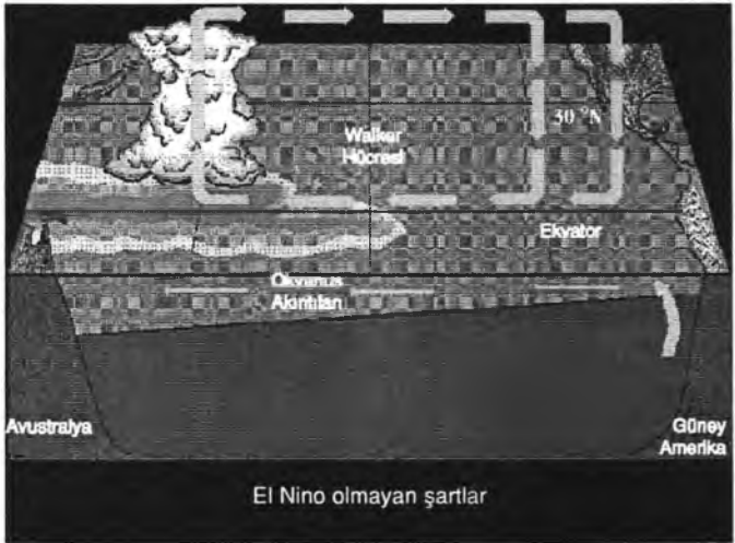
Şekil 2.15. El Nino olmayan (La Nina) yıllarında Avustralya ile Güney Amerika kıyıları arasındaki okyanus akıntıları, upwelling, Walker dolaşım hücresi ve batı Pasifik’te oluşmuş sıcak su havuzu ile birlikte konvektif fırtına bulutları gösterilmektedir.
