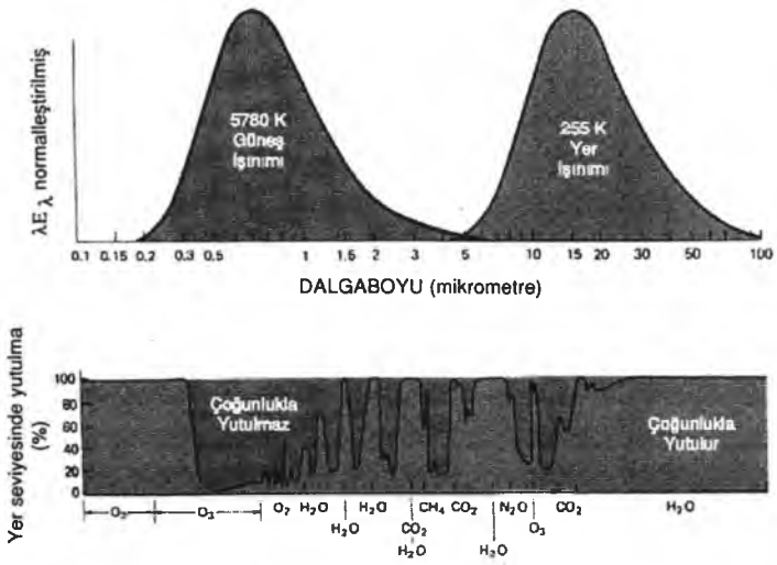
Şekil 1.10. Güneş ışınımı daha çok kısa boylu dalgalarla gelir ve atmosferden kolayca geçer. Dünya yüzeyinden gelen ışınım ise uzun dalga boyludur ve Dünya atmosferindeki sera gazları tarafından büyük bir kısmı yutulur. Böylece atmosferin sera etkisi oluşur (Gedzelman, 1980).
