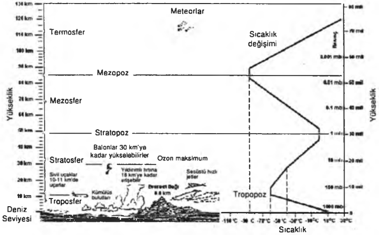
Şekil 1.2. Amerikan standart atmosfer tanımına göre sıcaklığın düşey değişimi ve atmosferin katmanları (Durmayaş ve Kadioğlu, 2001).
