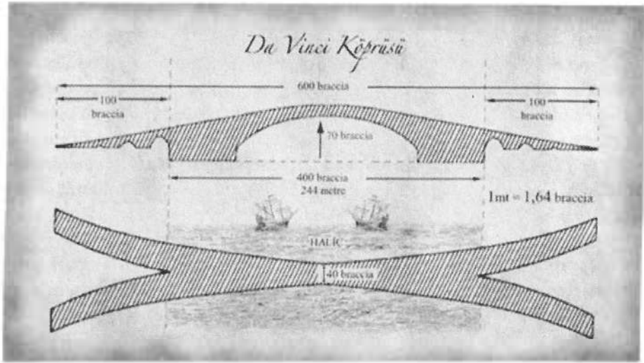
Da Vinci'nin Haliç köprüsü projesi
