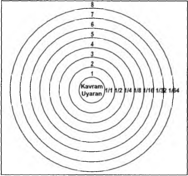
Şekil 16. Yüklemler Kümesi; hedef tahtası yöntemi
