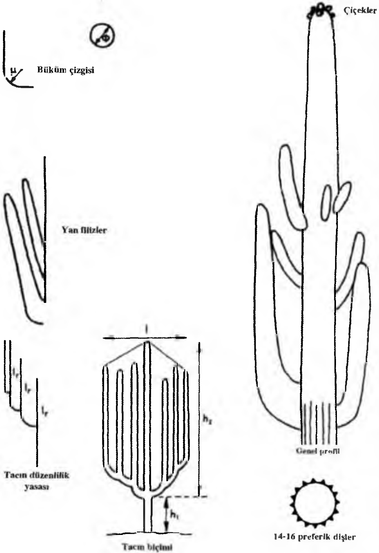
Şekil: 2- Candelaria kaktüsünün profilinin temel biçimsel birimleri (morphèmes)
