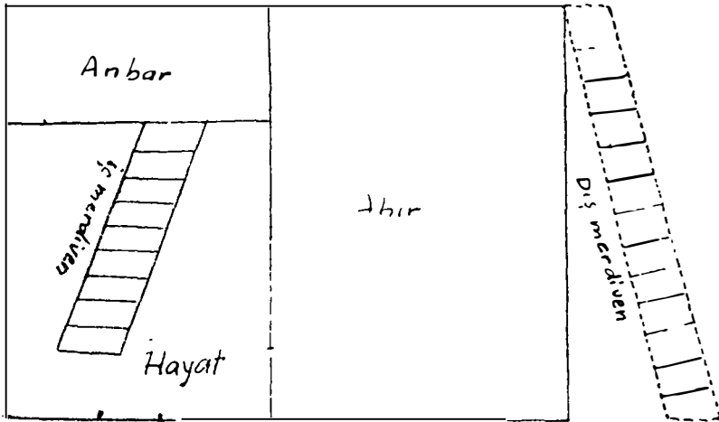
Şekil 7. Bir evin alt kat plânı.
