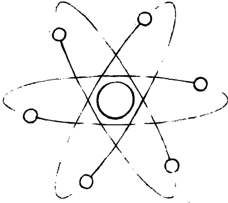
26.1 Rutherford'un Atomu
