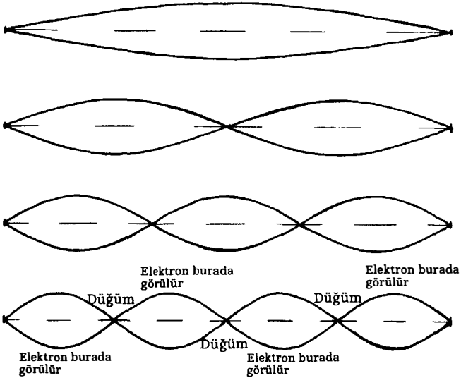
26.3 Einstein'ın Dalgaları
