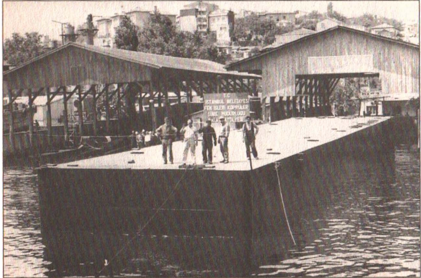
Duba atölyesinde imal edilen taşıyıcı duba, Galata Köprüsü'ne götürülüyor.
