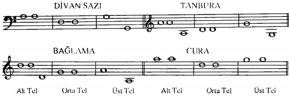
Şekil 3. Bağlama ailesinin LA sesine göre akortları
