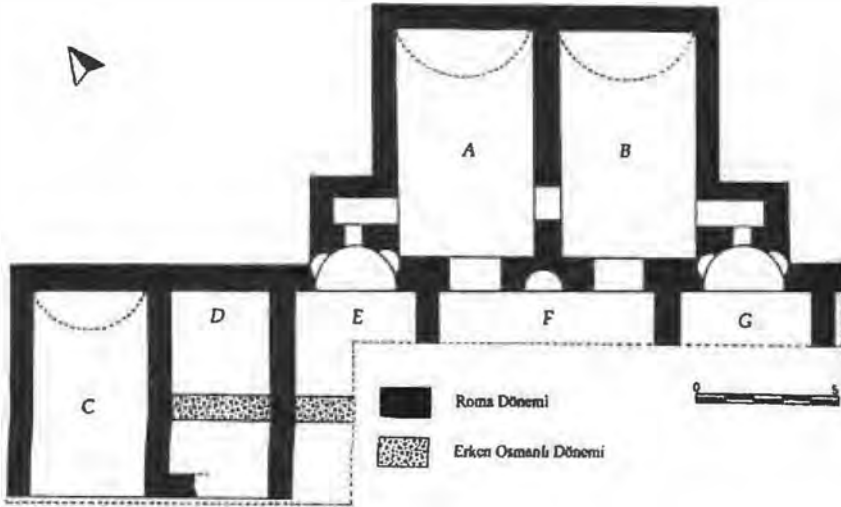
Çizim 1: Akropol II. Teras Tonozlu Mekânlar Taban Planı
