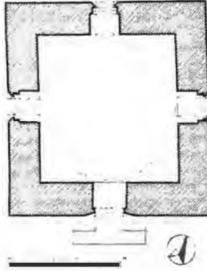
Şekil 1: Birgi, Aydınoğlu Mehmed Bey Türbesi Plânı (Ertan Daş'tan)
