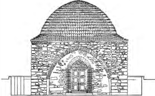
Şekil 9: Batı Cephesi İçin Restorasyon Önerisi (2009, S. Bellibaş / Efes Kazıları).
