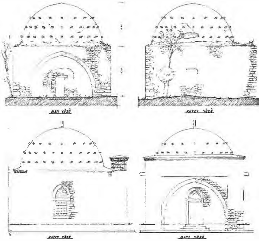
Şekil 7: M.Akok'un Türbeye İlişkin Rölöve Çalışması (üst) ve Restorasyon Önerisi (alt) (Vakıflar Genel Müdürlüğü Arşivi).
