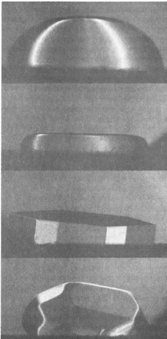
Resim 10: Soğudukça, helyum kristallerinin yüzleri daha belirgin hale geliyor.
