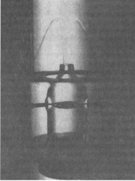
Resim 7. Fıskiye olayı, fotoğraf: J.F. Allen ve J.M.G. Armitage, 1971. J.F. Allen'in sonradan profesör olduğu St. Andrews Üniversitesi, Fizik ve Astronomi Okulu arşivinden.
