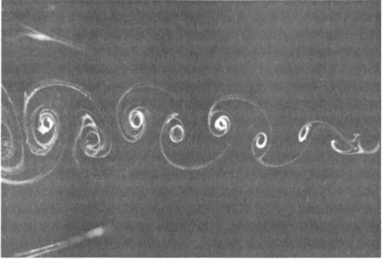
Resim 11. Yuvarlak bir engelin ardında akan bir sıvı, bir yandan diğerine değişken formda anaförler yaratır. Bu olay, teknelerdeki yelken iplerinde rüzgarın çıkarttığı ısıklı da meydana getiren olaydır. © ONERA
