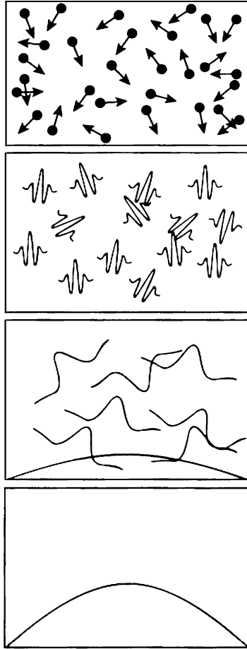
Resim 4. Wolfgang Ketterle'nin Einstein-Bose yoğunlaşmasını yorumlayışı. Yüksek sıcaklıkta gazın atomları her yöne gelişigüzel hareket eden titreşimli parçacıklardır. Sıcaklık düşerken, aynı atomların dalga benzeri karakterleri açıkça ortaya çıkar ve atomlar giderek artan biçimde dışa doğru etki alanlarını genişleterek üst üste çakışan dalga paketlerine dönüşürler. Sonunda, kritik sıcaklık T_C 'nin altına inildiğinde, ortak bir dalga formunda "yoğunlaşırlar." Mutlak sıfır noktasındaki atomlar, kendilerine has özellikleri kaybedip, tıpkı bir keman telinin bağlı iki ucu arasında yaptığı gibi, kutunun içinde büyük bir tek madde dalgası halinde titreşirler. Yukarıdan aşağıya doğru yüksek sıcaklık ( T \gg T_C ) ve düşük sıcaklık T = T_C , T = 0 olarak düşünülmüştür.
