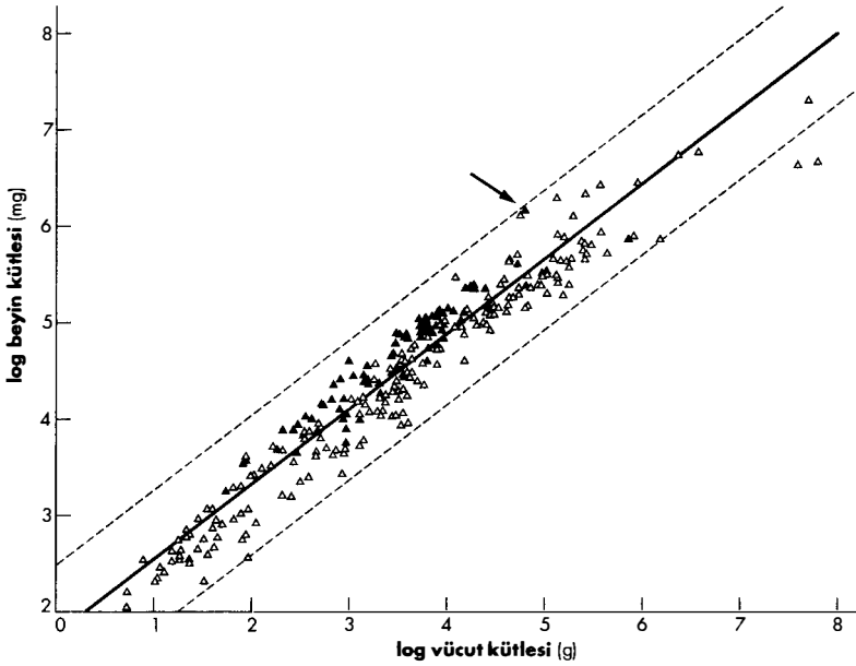
3. Plasentalı memelilerin farklı türleri için vücut kütlelerine göre beyin kütlelerinin log-log grafiği; içi dolu üçgenler primatlardır. Martin'den uyarlandı [bkz. Kaynakça].
