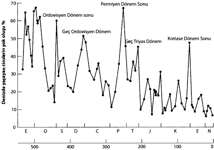
Fanerozoik Üstzaman boyunca denizde yaşayan cinslerin yok oluş yüzdesi. Sepkoski'den uyarlandı [bkz. Kaynakça].
