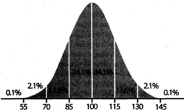
Şekil 1 İstatistikî IQ dağılımı grafiği. Kaynak: Wikipedia
