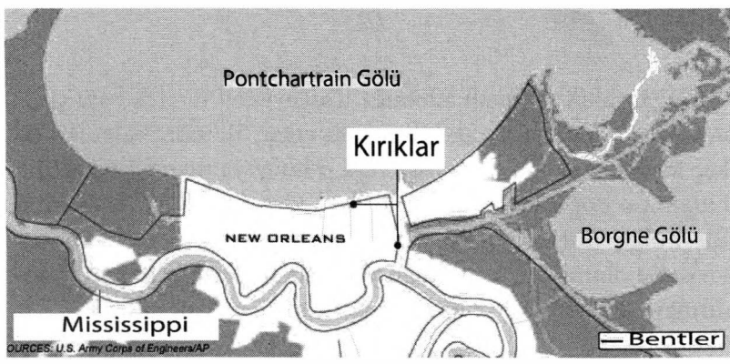
Şekil 2 New Orleans şehrini koruyan bentler ve bunların Katrina Kasırgası esnasında kırıldığı iki yeri gösteren harita.
