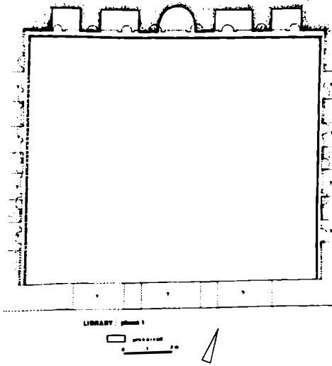
Lcv. XVI, Res. 1: Neon Kütüphane Yapısı, 1. evre planı (M. S. 120 sonrası), (M. Waelkens, aynı eser, s. 401, Fig. 7).
