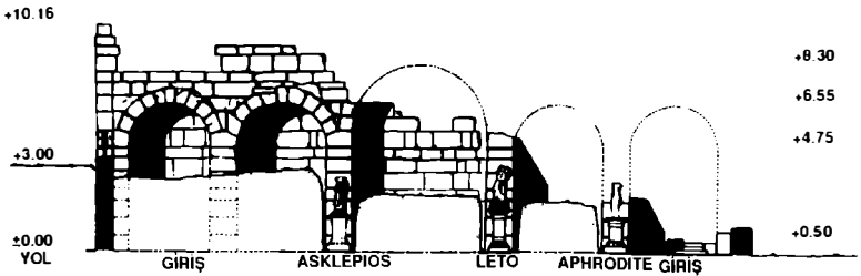
Lev. XIV, Res. 1: Kremna Kütüphanesi yapısı kesiti (J. Inan, 1970 Kremna Kazısı Raporu, Lev. VIII).
