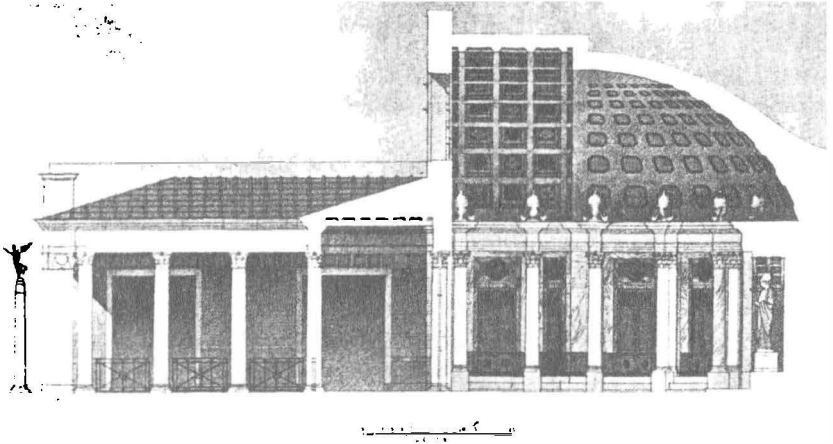
Ler. IX, Res. 1: Timgat Kütüphanesi, kesit [C. Callmer, aynı eser, s. 181, Res. 23].
