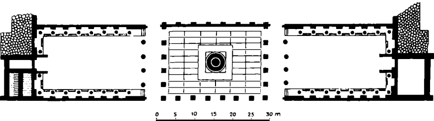
Lev. VII, Res. 3: Roma Ulpia Kütüphanesi kesiti (C. Callmer, aynı eser, s. 163, Res. 9).
