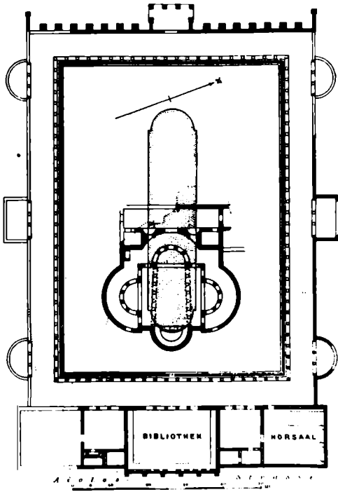
Ler. XXV, Res. 2: Atina'da Hadrian Stoa'sı ve Kütüphanesinin planı (W. Judeich, Topographie von Athen , s. 376, Res. 49).
