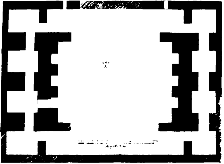
Lev. XXIII, Res. 2: Nysa Kütüphanesi, birinci kat planı (W. v. Diest, Nysa ad Meandrum , Lev. VIII).
