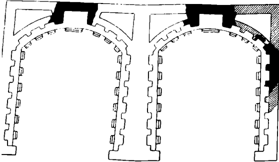
Lev. VI, Res. 2, 3: Roma'da Palatinus Apollon Tapınağı Kütüphanesinin planı ve apsisin kesiti (C. Callmer, aynı eser, s. 158, Res. 6-7).
