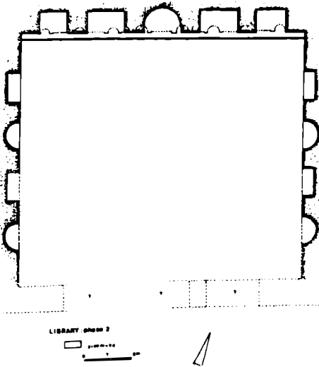
Lev. XVI, Res. 2: Neon Kütüphanesi Yapısı, 2. evre planı (II. yy. sonu). (M. Waelkens, aynı eser, s. 404, Fig. 12).
