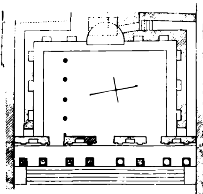
Lev. X, Res. 1: Heberdey'e göre Ephesos Kütüphanesinin kesiti (R. Heberdey, Vorläufiger Bericht über die Grabungen in Ephesos, s. 63-64, Şek. 16).
