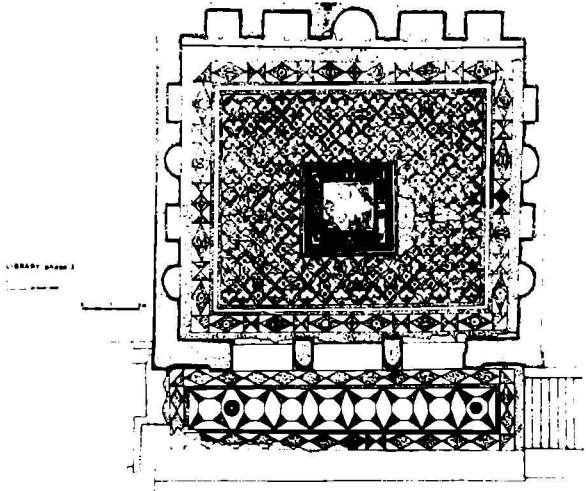
Ler. XVII, Res. 2: Neon Kütüphanesi, 3. erre yapısı planı (M. Waelkens..., aynı eser, s. 404, Fig. 13).
