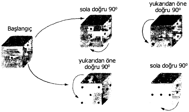
Şekil 4: Bir zarın önce sola doğru 90 derece, ardından yukarıdan öne doğru 90 derece döndürülmesiyle gelen yüz, bu sıra tersine çevrildiğinde bulunan yüzden farklıdır.
