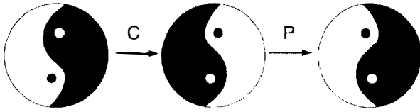
Şekil 9: Yin Yang sembolünün, negatifinin ayna görüntüsüyle karşılaştırılması.
