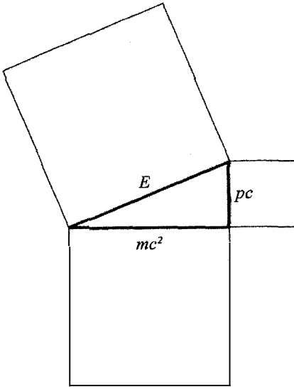
Şekil 2: Einstein, enerji ve Pisagor teoremi. Einstein'ın görelilik kuramında hareket halindeki bir cismin enerji miktarı E , tabanı bu cismin duran haldeki enerjisinin büyüklüğüyle ( mc^2 ) orantılı olan bir diküçgenin hipotenüsünün karesinin alanıyla ve cismin, momentum ve ışık hızının çarpımıyla orantılı olan hareket enerjisi pc 'yle orantılıdır.
