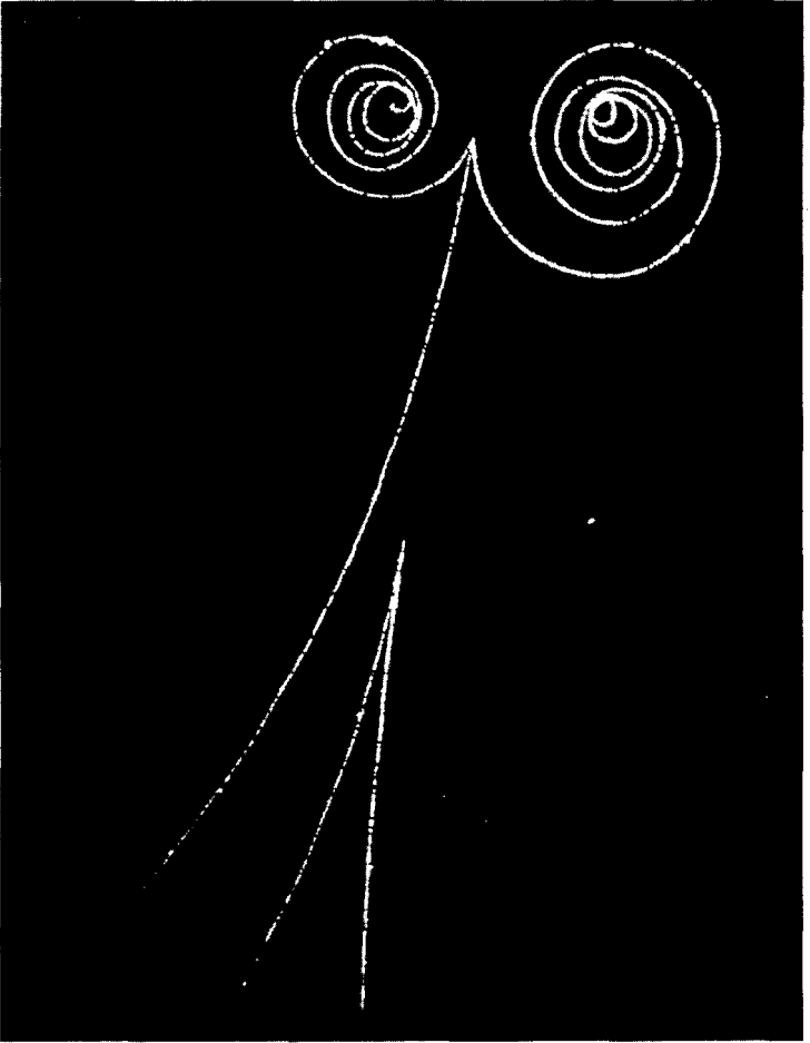
Şekil 6: Bir elektron ve bir pozitronun oluşumu. Yüksek enerjili bir kozmik ışın bir elektronu atomun dışına fırlatmış –görüntünün üst kısmından sol alta uzanan yumuşak eğimli yol bunun izi. Bir elektron ve bir pozitron oluşturmaya da yetecek enerji mevcut, görüntünün üst bölümünde, dar kıvrımların meydana getirdiği spiraller bunlara ait izler. Resmin alt kısmında bir elektron ve pozitron daha oluşup, ters dönmüş V izini bırakarak birbirlerinden ayrılmışlar.
