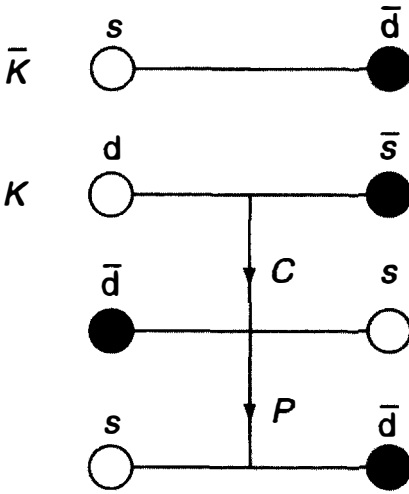
Şekil 10: Jekyll ve Hyde K^0 . d (down/aşağı) ve s (strange/acayip) kuarklar ve anti-kuarklardan oluşan bir kaon ve antikaon (antikuarklar, simgelerinin üzerindeki düz çizgiyle belirtiliyor). C'nin (kuarkın "negatif görüntüsü" olan antikuarka dönüşmesi) ve P'nin (ayna tersi) etkisi gösteriliyor. Etki itibarıyla kaon antikaona dönüşmüştür.
