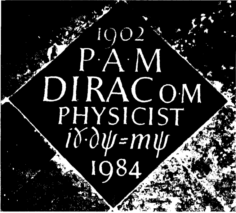
Şekil 3: Westminster Kilisesi'nde Dirac için dikilen ve üstüne onun denklemi yazılan mezar taşı. y simgesi Ek 2: "Dirac Kodu" içinde tarif edilen "gama" matrislerini ifade ediyor.
