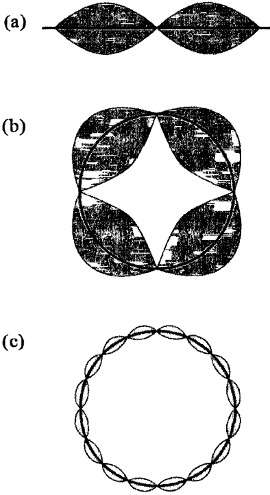
Şekil 1: Dalgalar var olabilmek için çembere tam olarak sığmak zorundadır.
