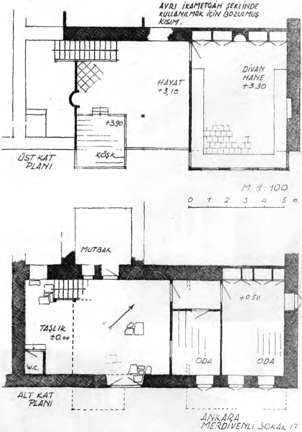
31. Merdivenli sokak 17 - Ankara. Pencere ve plân, zamanla tadile uğramıştır. Hayat ve köşkü karakteristiktir.
