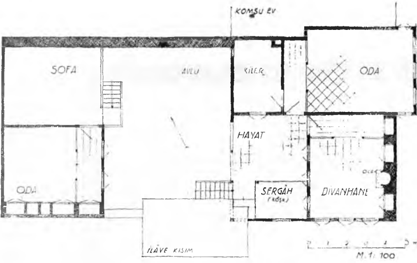
35. Üst kat plânı
