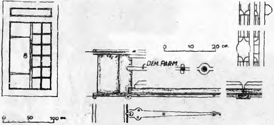
118. Erzurum mahallesi Erzurum sokak 60 - Ankara (Sofaya bakan bir oda penceresi detayı:)
