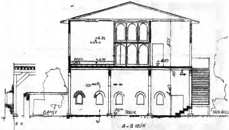
71. Müftü A. Halim Efendi konağı kesiti - Ankara
