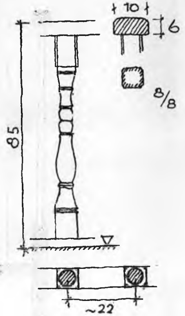
127. Bir Ankara evinde sofa kenarı parmaklığı detayı.
