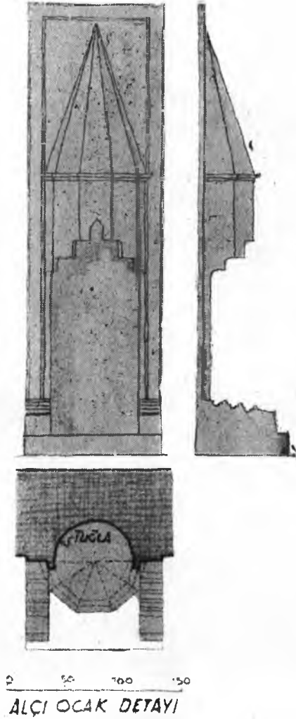
129. Erzurum mahallesi Erzurum sokak 60 - Ankara Alçı ocak detayı.
