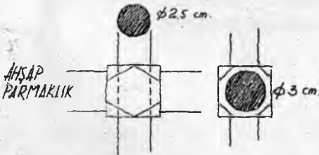
120. Ankara evinde çıkma konstrüksiyonu, pencere, parmaklık ve kapak detayı
