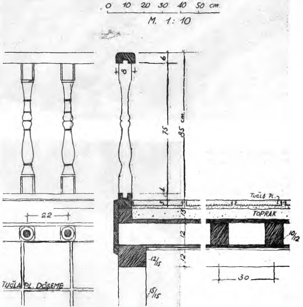
88. Hamamönü, Göztepe sokak 27 numaralı evin sofa parmaklığı ve döşeme detay kesiti
