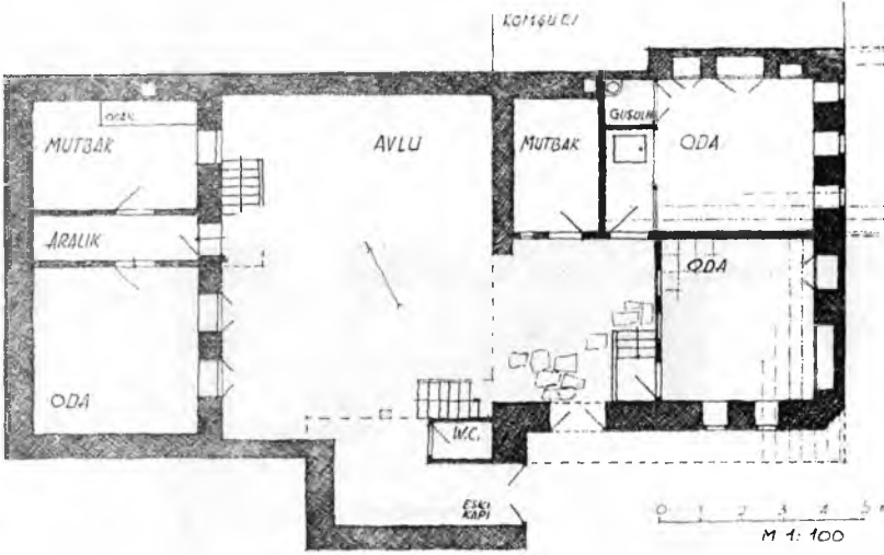
36. Alt kat plânı
