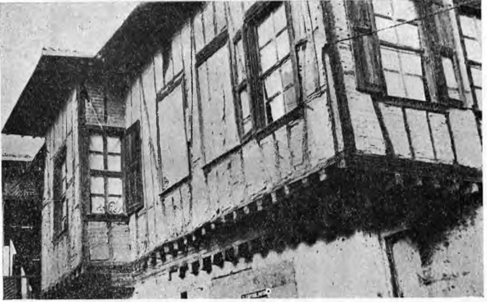
77. Diğer bir hususi çıkma şekli
