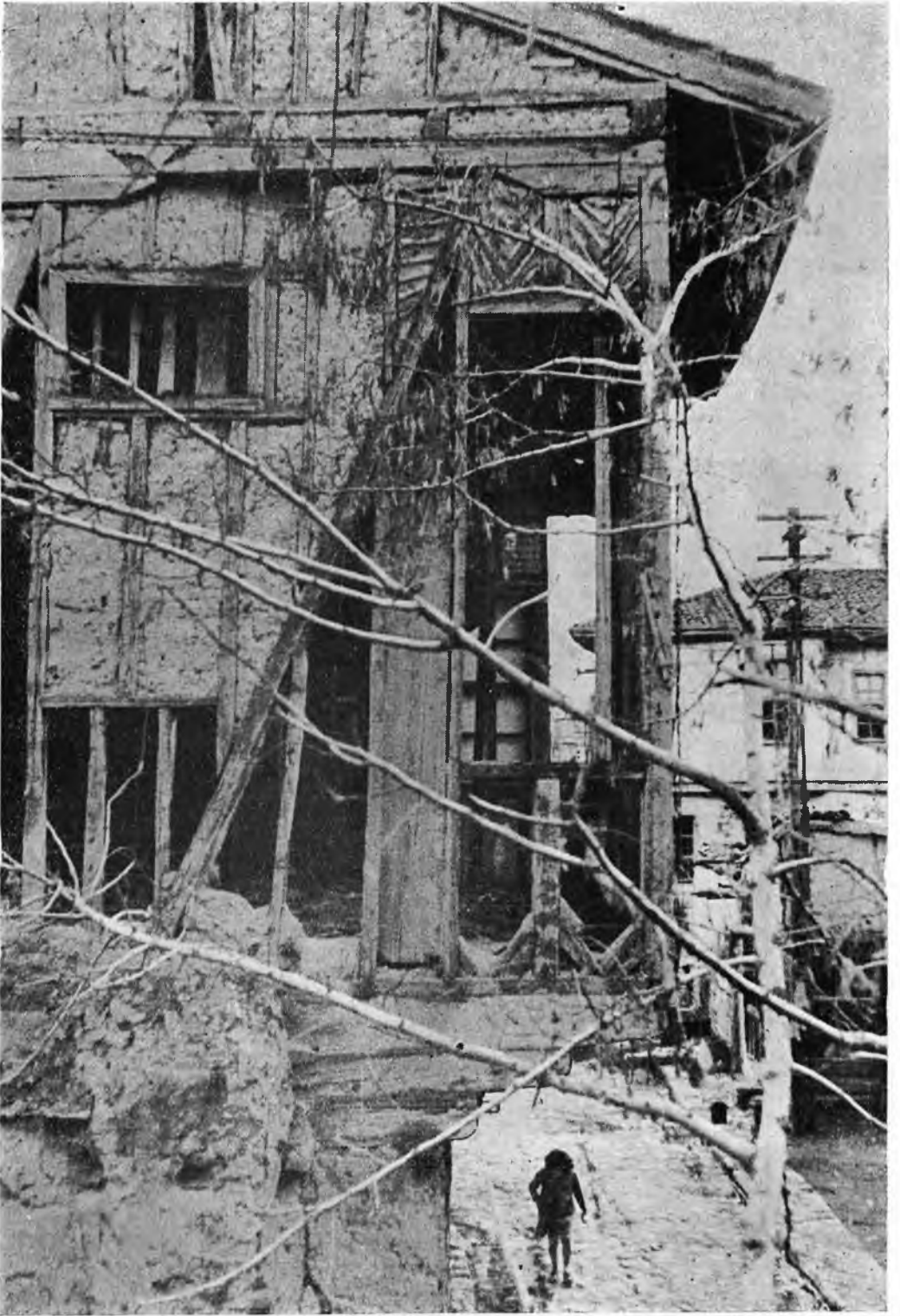
75. Aynı evden diğerk bir detay fotoğraf (Çıkma kirişlerine gelen yük, payandalarla taşıyıcı duvarlara aktarılmak suretiyle, hafifletilmiştir.)
