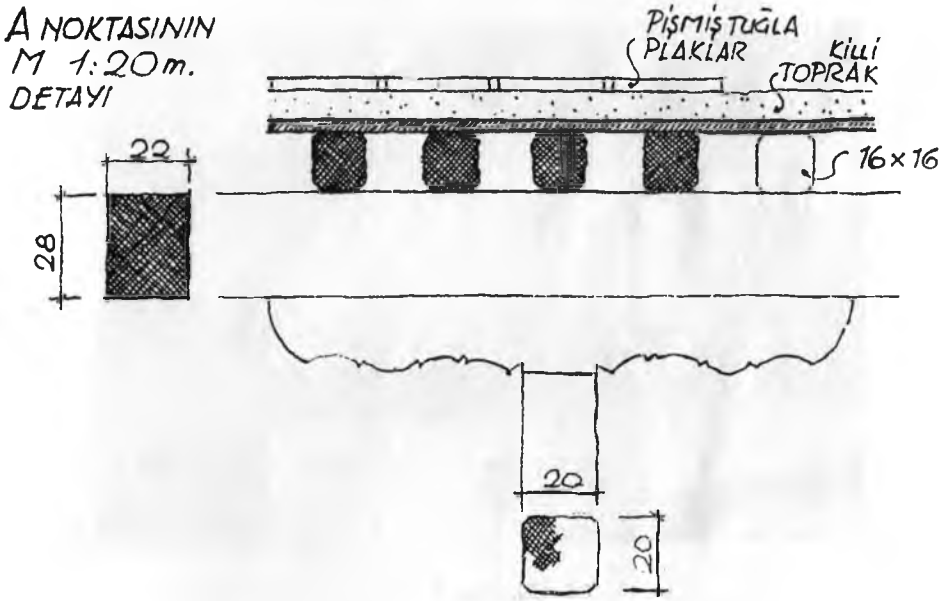
87. Müftü Abdülhalim Efendi konağında bir direk başlığı ve döşeme konstrüksiyonu detayı - Ankara
