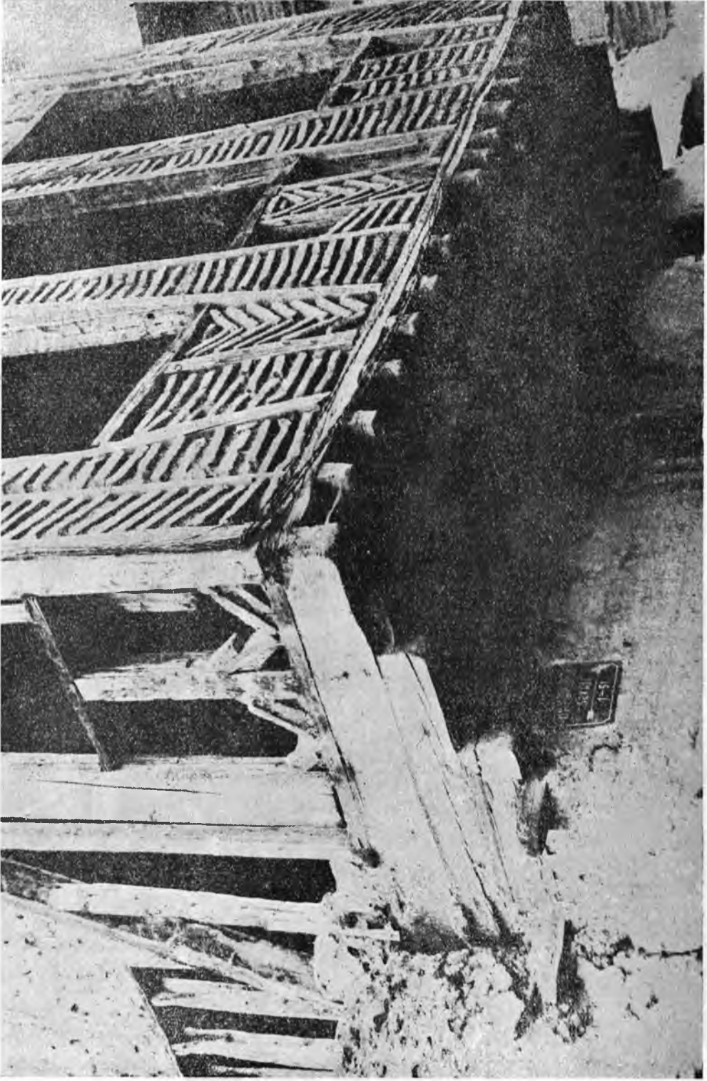
74. Ankara evinde orijinal bir çıkma konstrüksiyonu - Hamamönü, Ankara
