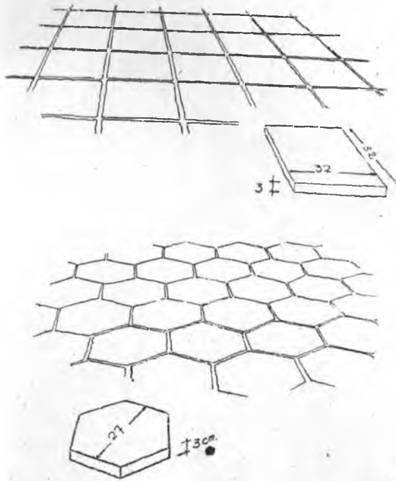
130, 131. Kare ve altı köşeli pişmiş tuğla plâklı döşemeler
