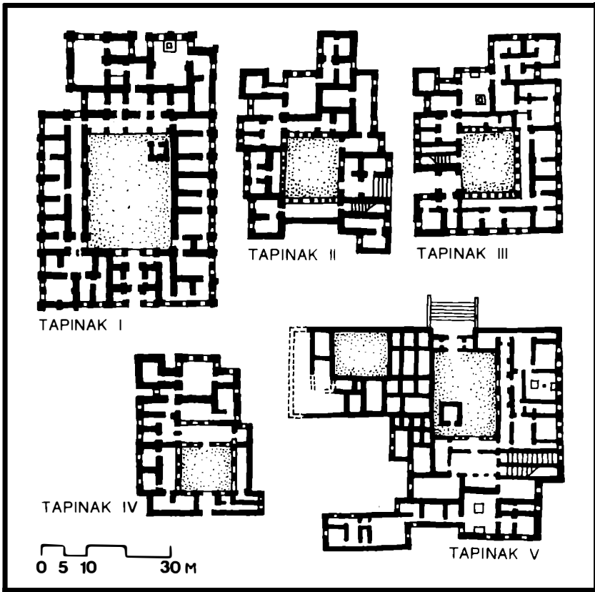
Şekil 50. Hattuşa'daki beş tapınağın planları
