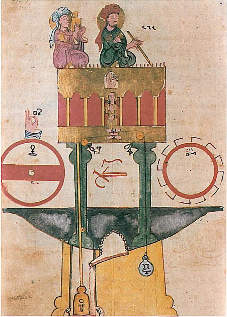
Resim: 129- El-Cezeri'nin Kitâb fî Mârifet el-Hiyâl el-Hendesiye (Otomata) albümünden tepesinde iki yazıcı oturan otomatik kan ölçęęi (hastadan alınan kan miktarını ölçer) (1206, Diyarbakır) (İstanbul Topkapı Müzesi Kitaplığı, 3472, s. 133a) Mechanical basin with two scribes for measuring the exact amount of blood taken from the patient, from the Automata of al-Jazari "Kitâb fî Mârifet al-Hiyâl al-Handasiya" (Book of Knowledge of Ingenious Mechanical Devices), 1206, Diyarbakır (Library of the Topkapı Museum, Ahmet III, 3472, p. 133a).
