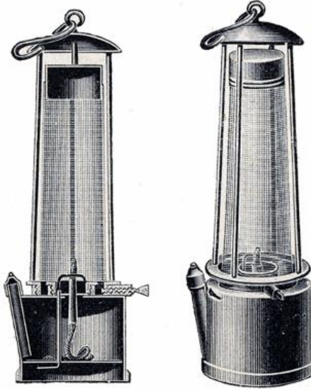
Fig. 192. Davy'sche Sicherheitslampe
