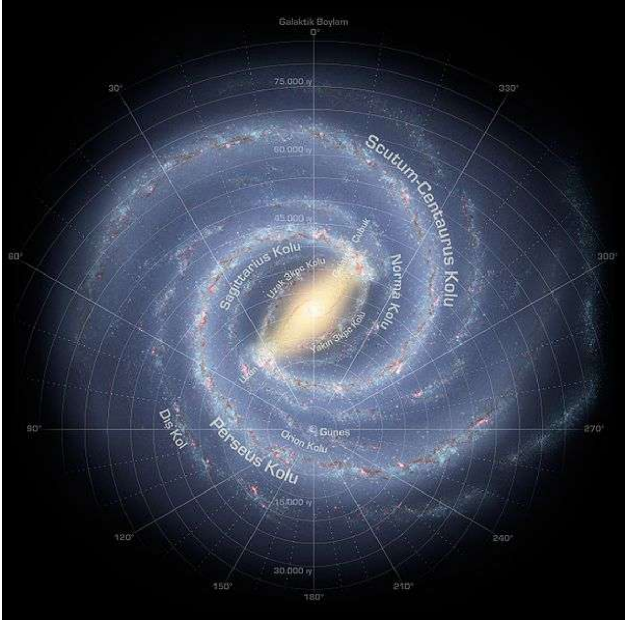
Samanyolu Galaksisi
