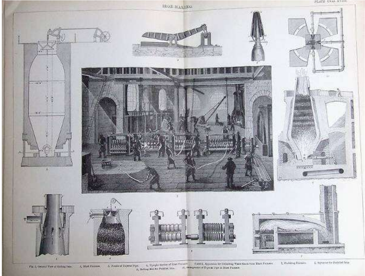
Kok kömürle Demir Fırını
