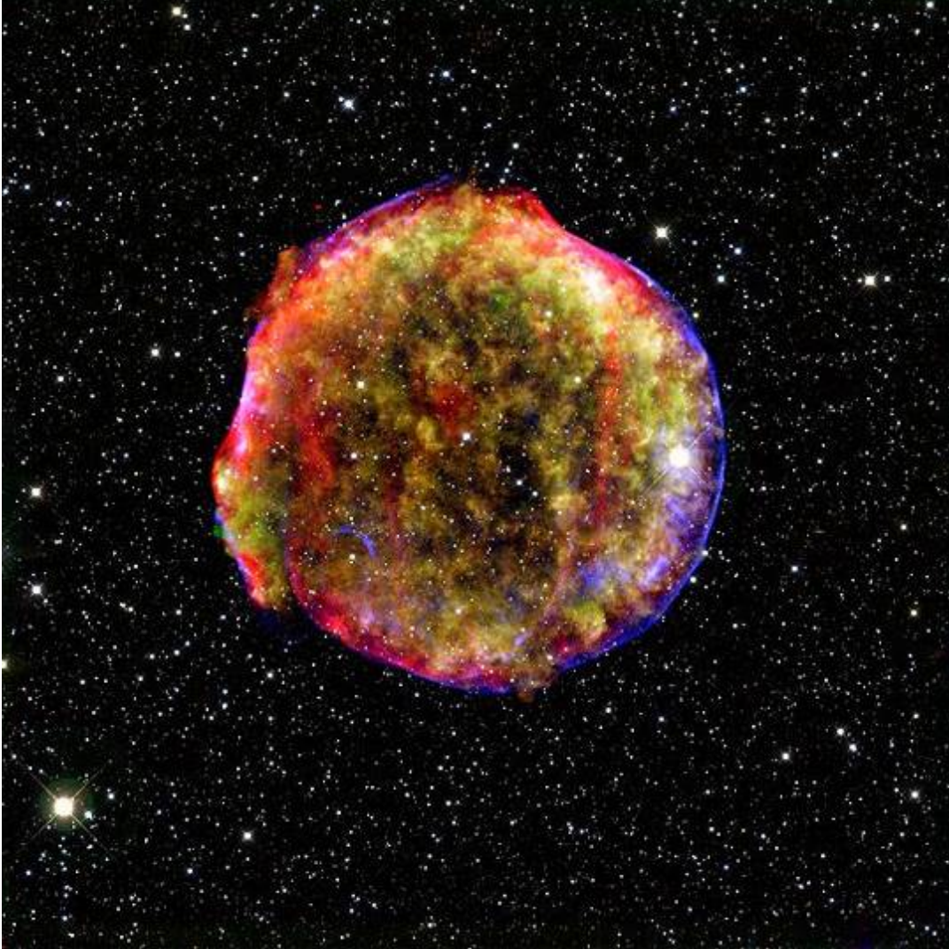
Tycho Süpernovasının 4 asır sonraki resmi
