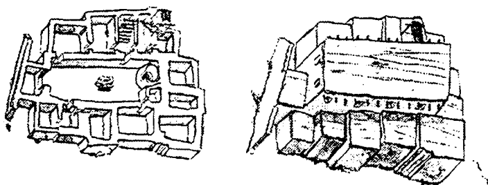
Üç parçalı planlı bir yapının izometrik planı (sol) ve rekonstrüksiyonu (sağ)
