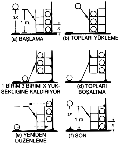
Şekil 4-2 Tersinir bir Makine
