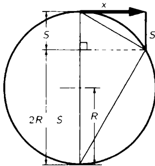
Şekil 5-4 İvme, çembersel yolun merkezine doğrudur. Düzlem geometriden x/S = (2R - S)/x \approx 2R/x 'dir; burada R dünyanın yarıçapı (6437 km), x bir saniyede "yatay olarak gidilen" mesafe ve S bir saniyede "düşülen" mesafe (4,9 metre)dir.
