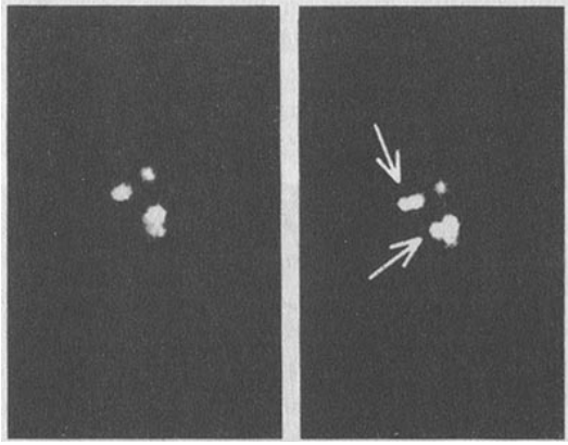
Şekil 5-12 Yeni yıldızların oluşumu?
