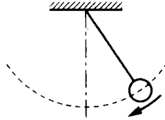
Şekil 4-7 Basit sarkaç
