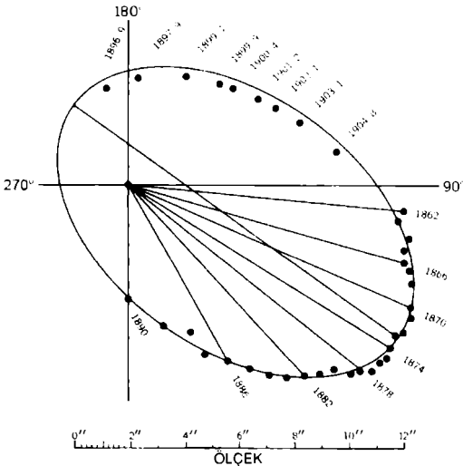
Şekil 5-7 Sirius B yıldızının Sirius A 'ya göre yörüngesi.
