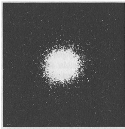
Şekil 5-8 Bir küresel yıldız kümesi.
