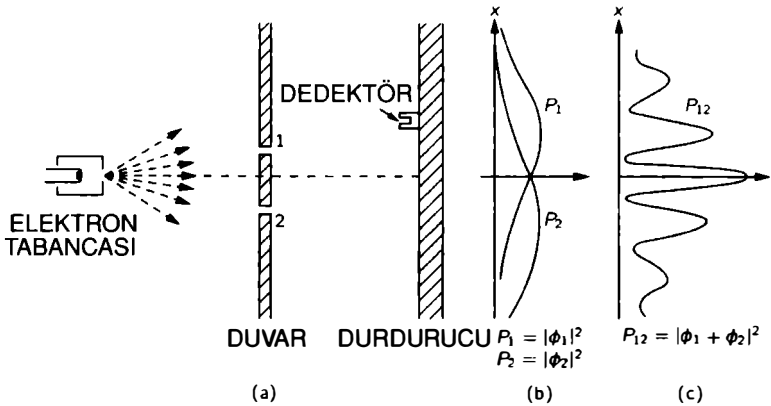
Şekil 6-3 Elektronlarla girişim deneyi
