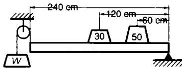
Şekil 4–6 Bir ucundan destekli ağırlık yüklü çubuk
