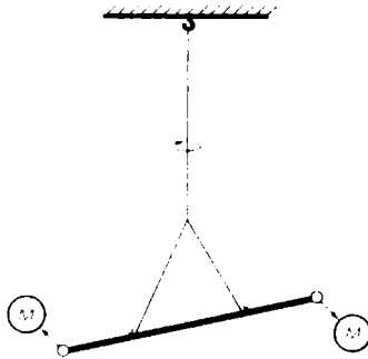
Şekil 5-13 Küçük cisimler için evrensel kütleçekim yasasını doğrulamak ve G kütleçekim sabitini ölçmek için Cavendish tarafından kullanılmış olan düzeneğin basitleştirilmiş bir diyagramı.
