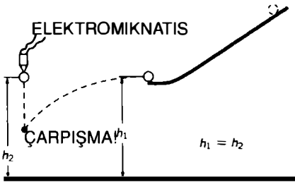
Şekil 5-3 Düşey ve yatay hareketlerin bağımsız olduklarını gösteren düzenek.
