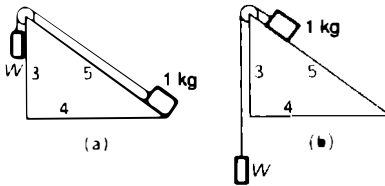
Şekil 4-3 Eğik Düzlem
