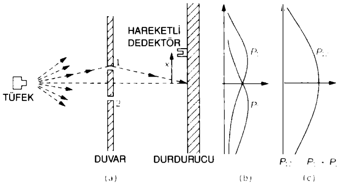
Şekil 6-1 Mermilerle girişim deneyi
