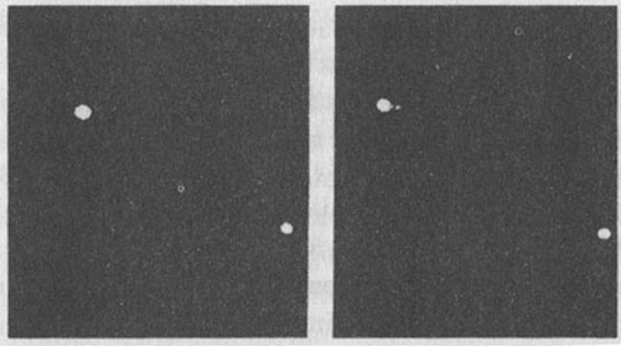
Şekil 5-6 Bir çift yıldız sistemi.
