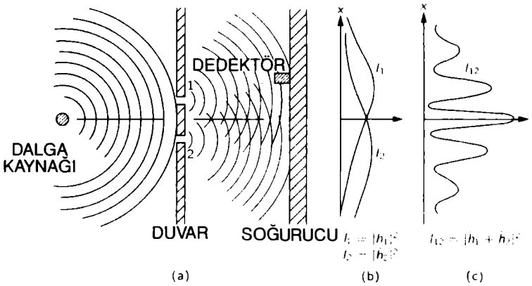
Şekil 6 - 2 Su dalgalarıyla girişim deneyi
