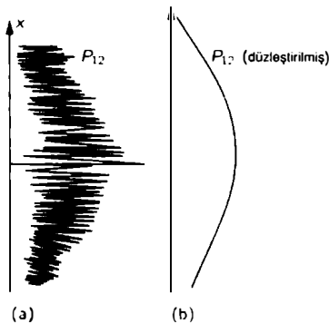
Şekil 6-5 Mermilerle-girişim deseni (a) gerçek (şematik), (b) gözlenen
