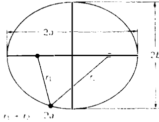
Şekil 5-1 Elips
