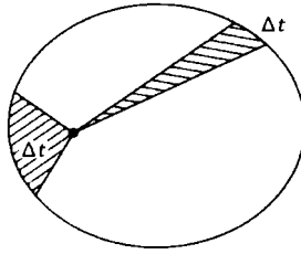
Şekil 5-2 Kepler'in alanlar yasası.
