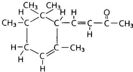
Şekil 1-10 Resimdeki madde \alpha -irone (süsen özü).
