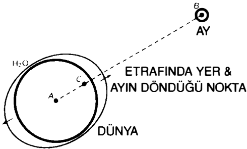
Şekil 5-5 Gel-gitli dünya-ay sistemi.
