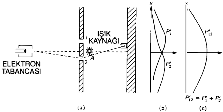
Şekil 6-4 Farklı bir elektron deneyi
