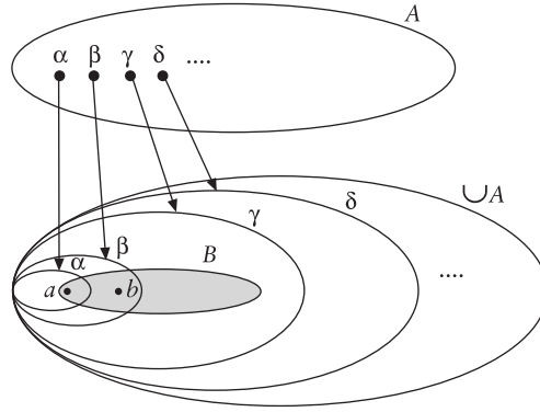
A, ordinaller kümesi. Aslında şekil yanlış, çünkü, örneğin, \alpha, \beta 'nin bir elemanı olmalıydı. Doğru şekil kafa karıştırıcı demeye cesaret edemeyiz de, çok karmaşık.
