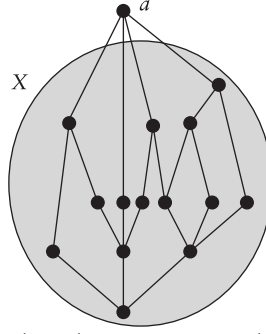
Sıralanmış bir X kümesinin tepesine bir eleman eklemek
