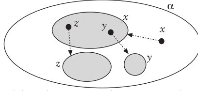
\in -kapalı bir \alpha kümesi: \alpha 'nın her ögesi \alpha 'nın bir altkümesi
