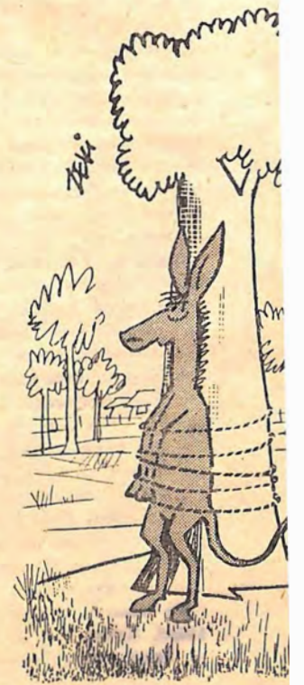
— Bu defa da ipi ko
