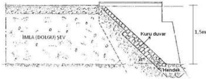
Şekil 1: Kanal Şevi
