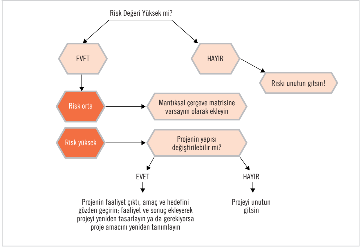
Çizim 11.1 Risk değeri yüksekse izlenecek algoritma
