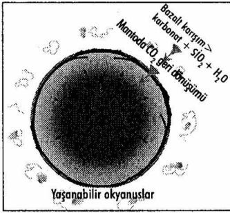
Şekil 62. Okyanusların oluşumunda dördüncü aşama; 4,26-3,90 milyar yıl önce, yaşanabilir okyanusların ortaya çıkışı. Yüzey sıcaklığı 55-105 °C.
