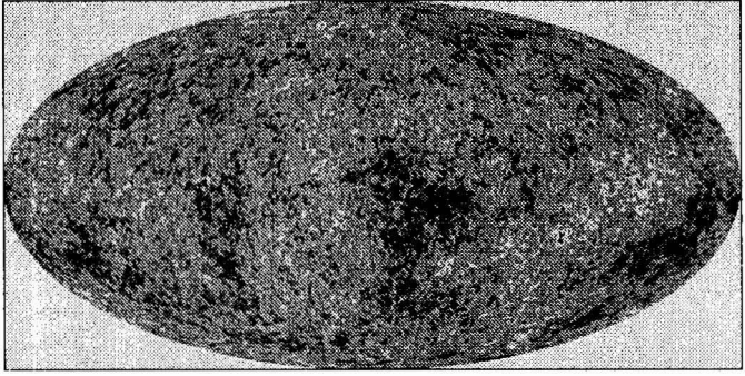
Şekil 48. WMAP Uydusu (Wilkinson Microwave Anisotropy Probe - Wilkinson Mikrodalga Anizotropi Sondası), tüm gökyüzündeki kozmik mikrodalga ardalan ışınlamadaki sıcaklık dalgalanmalarını, derecenin 100.000'de 1'i hassaslığıyla ölçebiliyor. Evrendeki ortalama sıcaklık 2,725 Kelvin (-270,275 °C). Şekildeki farklı tonlar, farklı ısı bölgelerini gösteriyor.
