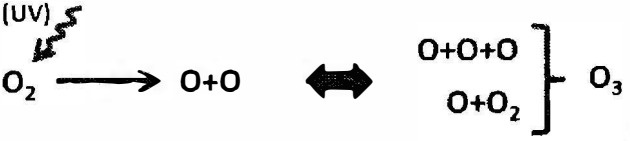
Şekil 102. Ozonun oluşumu.
