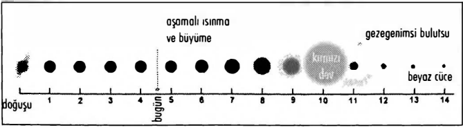
Güneş'in yaşamı (Büyüklikler ölçekli değildir)
