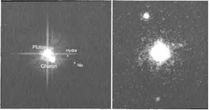
Solda Plüton ve üç uydusu ile sağda Haumea ve iki uydusu görülüyor.
