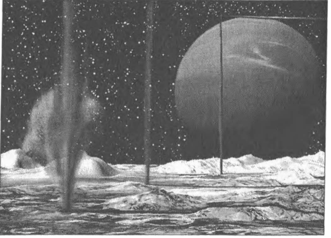
Triton'da 15 km kadar yükseğe azot püskürten gayzerler vardır.
