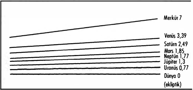
Gezegen düzlemlerinin ekliptik düzlemle yaptığı açılar.
