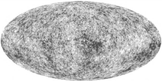
WMAP'in gözlediği kozmik mikrodalga arka plan ışıması haritası.
