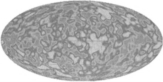
COBE'nin gözlediği kozmik mikrodalga arka plan ışıması haritası.
