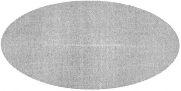
1964'te gözlenen kozmik mikrodalga arka plan ışıması haritası.
