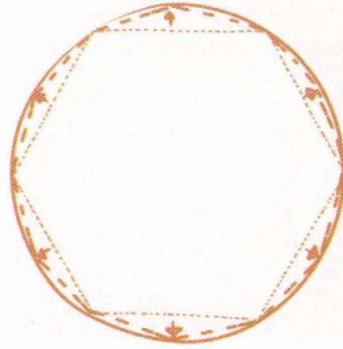
Resim Liu Hui'nin kendi daire oranı gösterimi.
