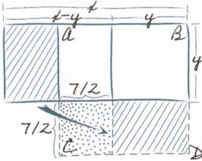
Çizim: Kareyi tamamlamak.
