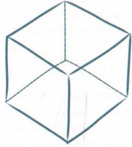
Çizim: Bir küpün 8 köşesi, 12 kenarı ve 6 yüzü vardır.
