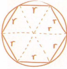
Resim Liu Hui'nin kendi daire oranı gösterimi.
