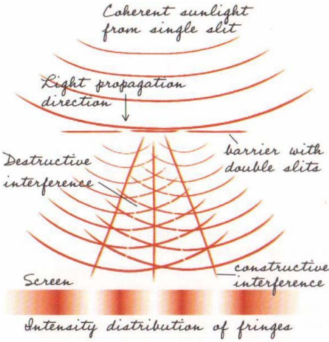
Çizim: Young'ın çifte yarık deneyi.
