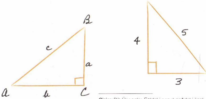
Çizim: Dik Üçgenler. Soldaki genel, sağdaki özel.
