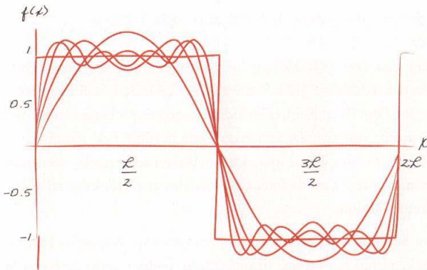
Grafik: Bir kare dalga ve sinüs dalgalarının sonlu toplamıyla yakınsamasını gösteren bir grafik. Yakınsama kare dalgaya doğru istendiği kadar ilerletilebilmektedir.
