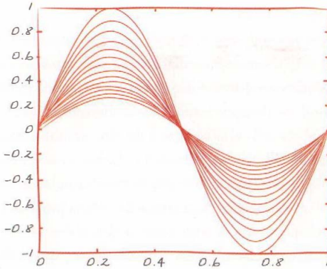
Grafik: Fourier'ın ısı denklemi çözümünde genliği zamanla azalan bir sinüs dalgası oluştuğu görülmektedir.
