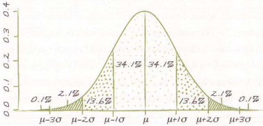
Grafik: \sigma ile gösterilen standart sapması klasik çan eğrisindeki alış satış farkının ölçüsüdür.
