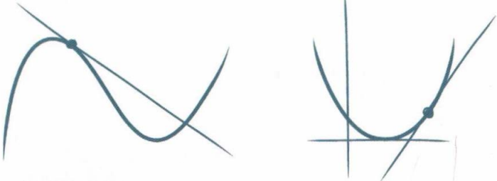
Çizim: Teğetler ve Eğriler.
