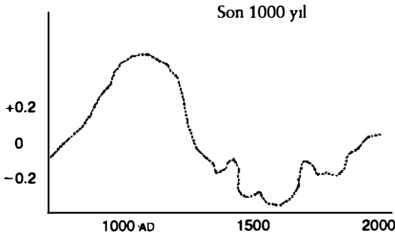
Şekil 2 Küresel sıcaklıklar
